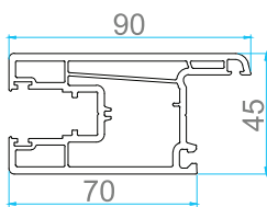
AP 305 SLIDING DOOR SASH
