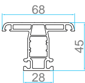
AP 706 CASEMENT T-MULLION
