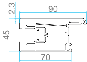
AP305 A SLIDING DOOR SASH
