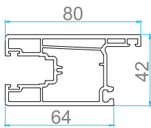
AP 105 SLIDING DOOR SASH
