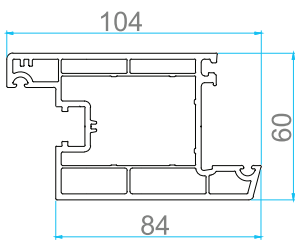
AP 215 INWARD DOOR SASH
