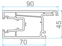
AP 305 SLIDING DOOR SASH
